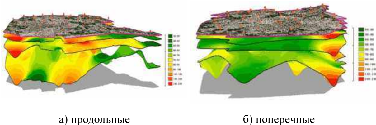
Рисунок 2. 3D карты распространения продольных и поперечных волн в городе Бухара
