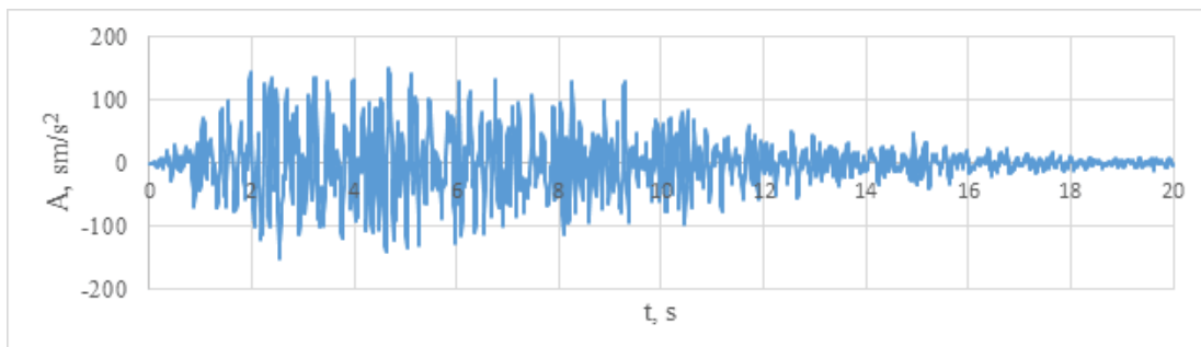
Рисунок 7. Синтетическая акселерограмма на основе среднего спектра, обобщающего реальные записи землетрясений
