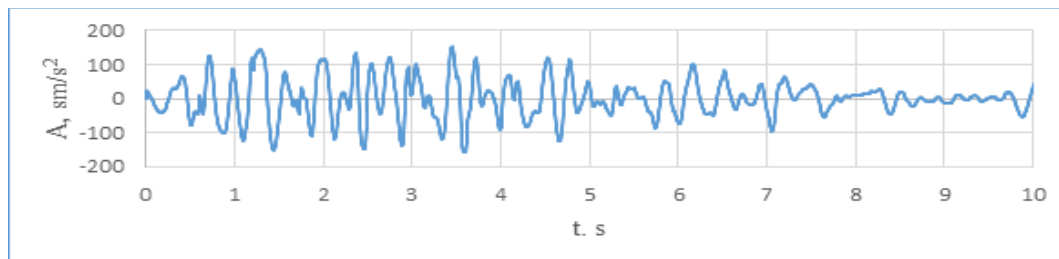
4-rasm. Ma'lum bir tezlanishga normalashtirilgan sintetik akselerogramma
