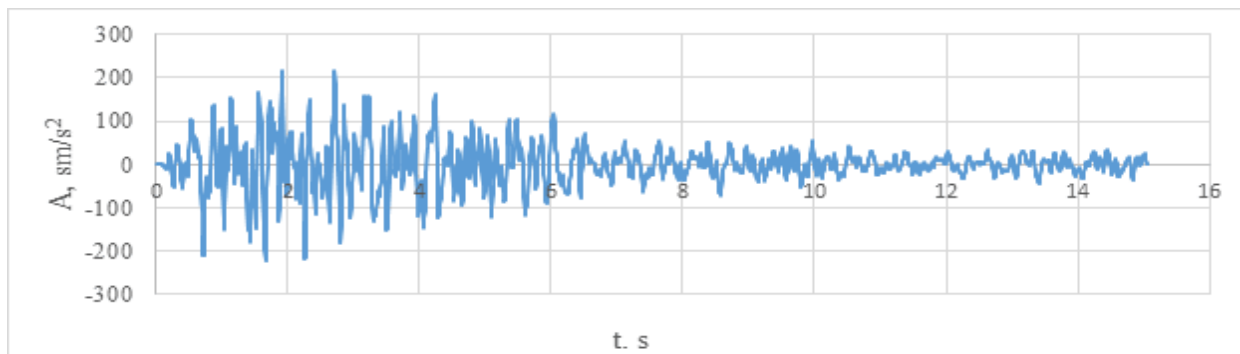
Рисунок 6. Синтетическая акселерограмма, созданная на основе спектра реакции грунта
