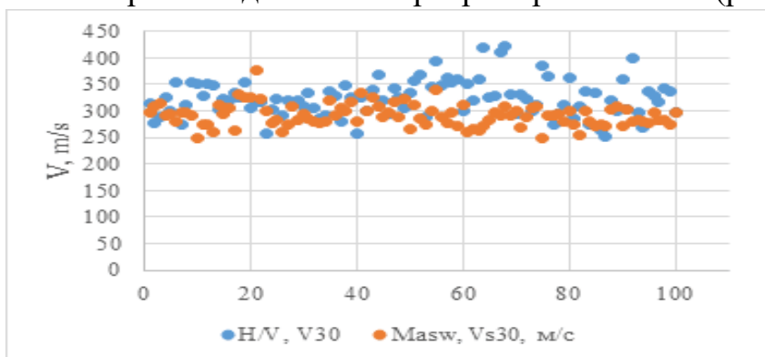
Рисунок 1. График скоростей, найденных методами микротремора и MASW (На примере района города Карши)
