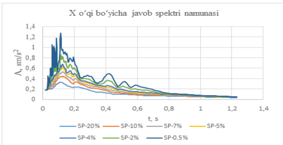
Рисунок 5. Спектры реакции различных законов затухания
