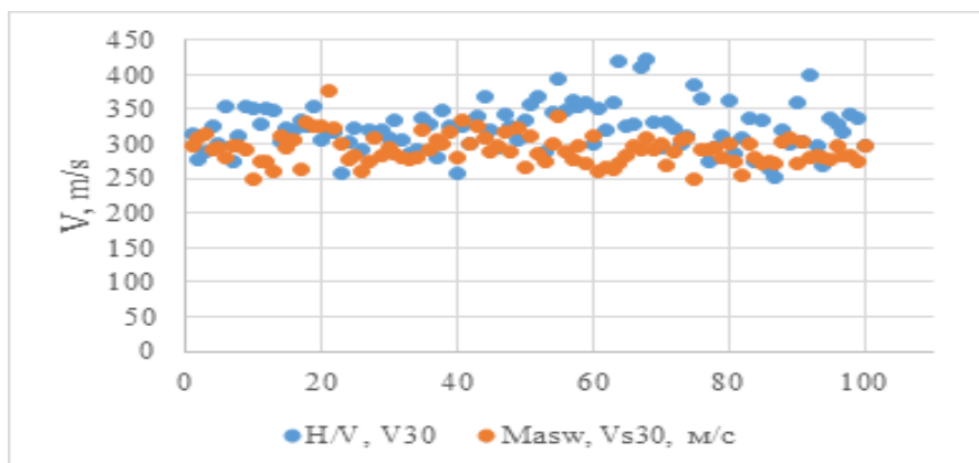
1-rasm. Mikrotremor va MASW usullar bilan topilgan tezliklar grafigi (Qarshi shahri hududi misolida)
