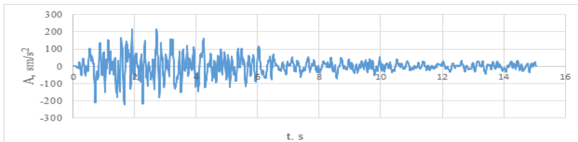
6-rasm. Grunt javob spektri asosida yaratilgan sintetik akselerogramma
