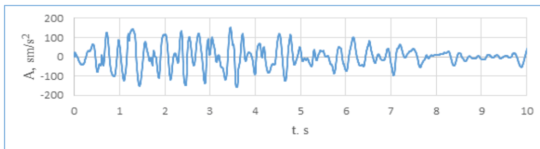
Рисунок 4. Синтетическая акселерограмма, нормированная к заданному ускорению
