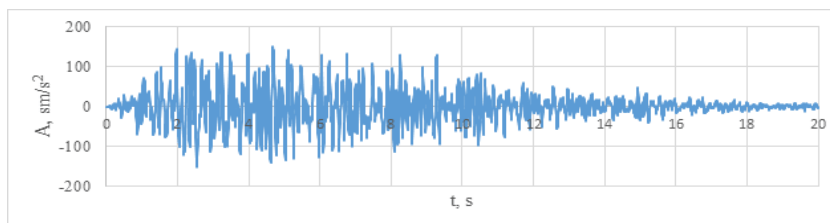
7-rasm. Real zilzila yozuvlarini umumlashtirib o'rta spektrga asoslangan sintetik akselerogramma
