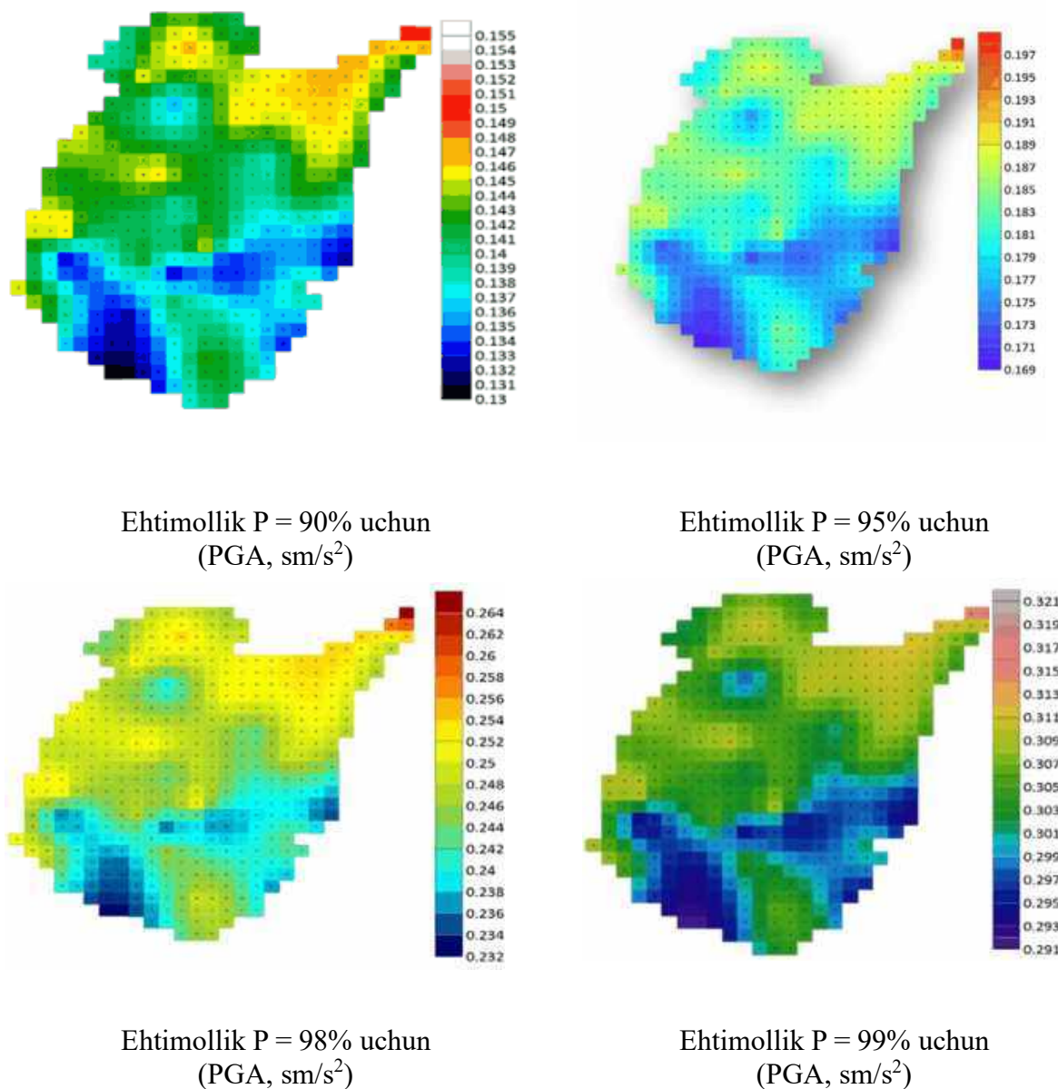
8-rasm. Buxoro shahri hududining turli xil grunt sharoitlarini hisobga olib yacheykalarga ajratilgan va o'rta spektrga asoslanib yaratilgan sintetik akselerogrammalar bazasi
