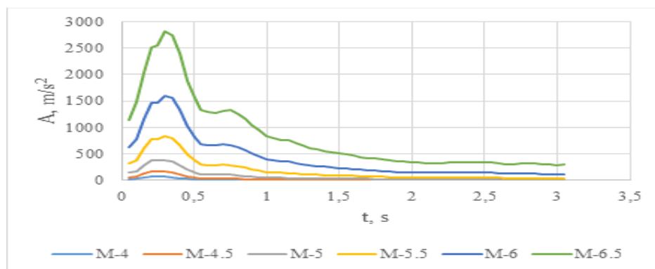
Рисунок 3. Спектр землетрясений разной магнитуды на одинаковом расстоянии
