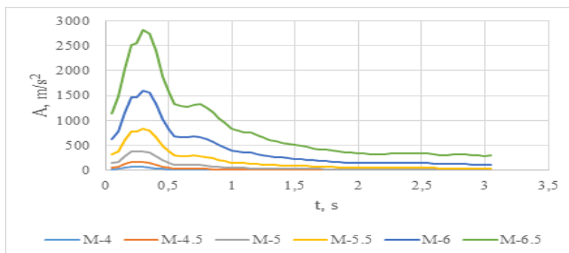
3-rasm. Bir xil masofada turli xil magnitudali zilzila spektri
