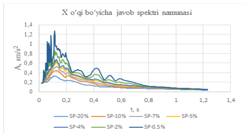
5-rasm. Turli xil so'nish qonuniyatlarining javob spektrlari
